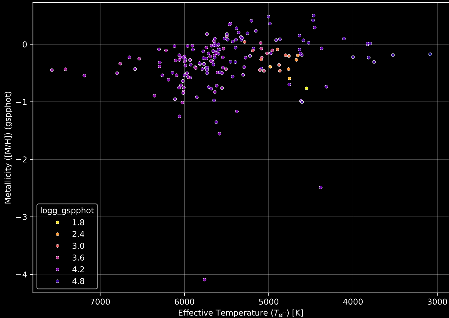
APOGEE DR17 Field: [115+71_MGA] Stellar Population Parameters (n= 180)
